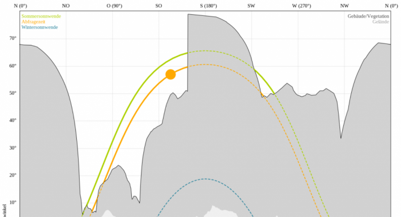
Sonnengang am 30.07.
